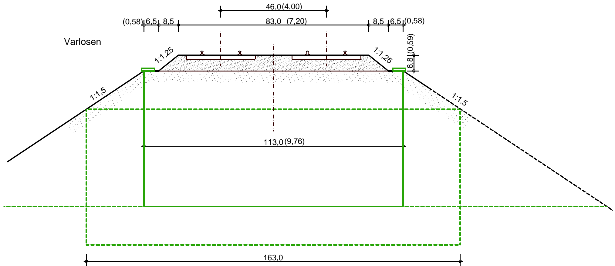
Maßstäblicher Schnitt durch einen Bahndamm in H0 (1:87)
