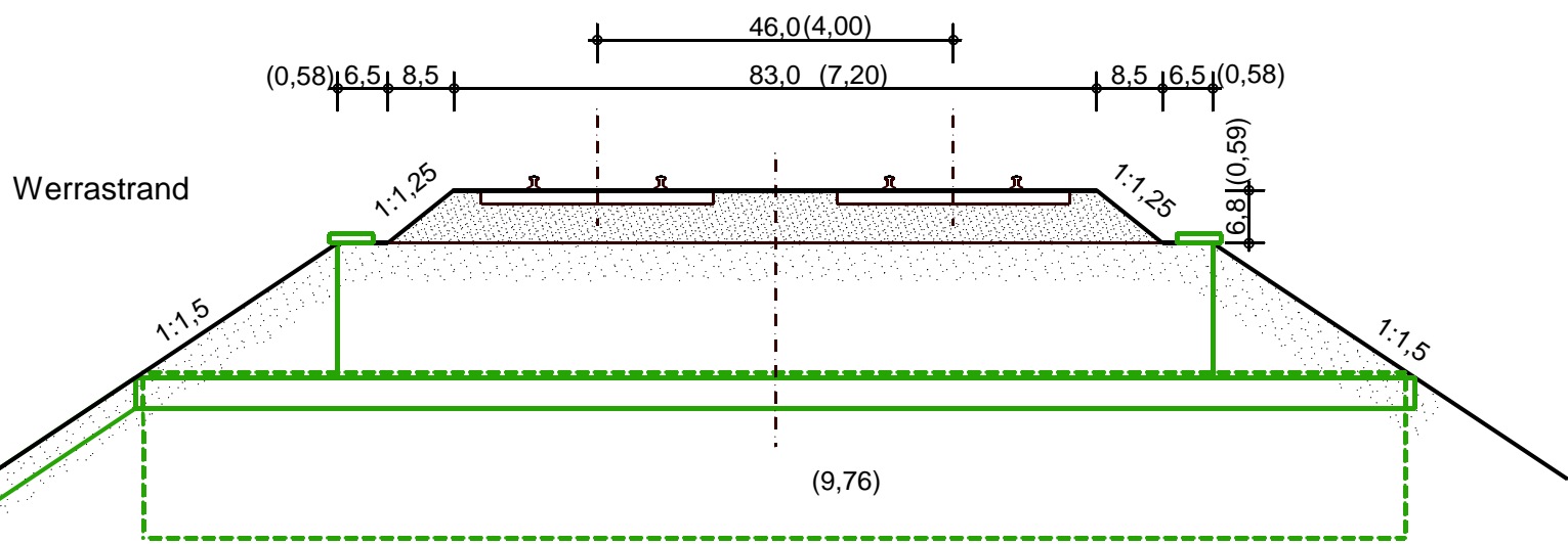
Maßstäblicher Schnitt durch einen Bahndamm in H0 (1:87)
