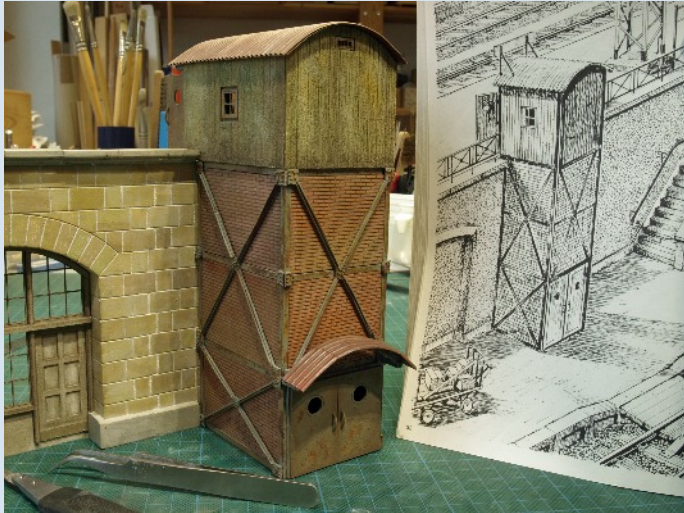
Der Lastenaufzug für Hochbahn- und Turmbahnhöfe kommt für H0 und Spur 0 und basiert auch auf einer Skizze von Pit Peg (†).
