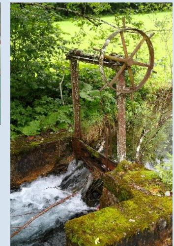
Mühlenwehr
